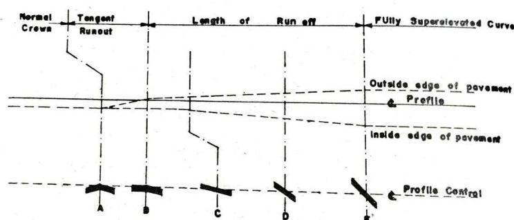
รูปภาพที่ ๔๑ การยกขอบทางโค้ง ใช้เส้นแบ่งครึ่งถนนเป็นจุดหมุน
