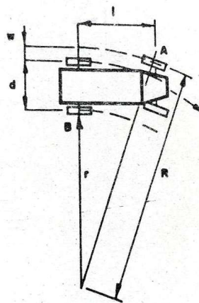
รูปภาพที่ ๔๖ รถเมื่อเข้าโค้งรัศมีขณะเข้าโค้งของล้อหน้ายาวกว่ารัศมีของล้อหลัง ที่มา: จิรพัฒน์ โชติกไกร. (๒๕๓๑).
