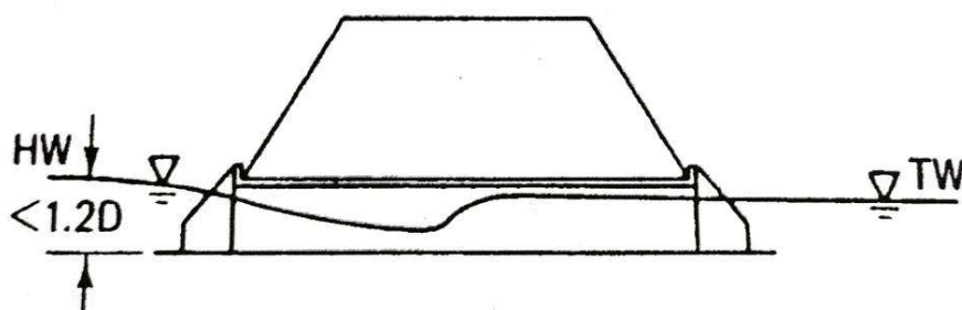
รูปภาพที่ ๕๘ ท่อลอดทางเข้าและทางออกไม่จมนเป็นการไหลในทางน้ำเปิด ที่มา: สำนักงานการปฏิรูปที่ดินเพื่อเกษตรกรรม.(๒๕๖๑).
