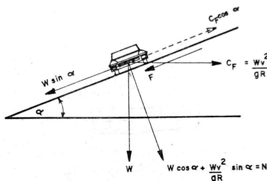
รูปภาพที่ ๔๐ การยกโค้ง ที่มา: จิรพัฒน์ โชติกไกร. (๒๕๓๑).
