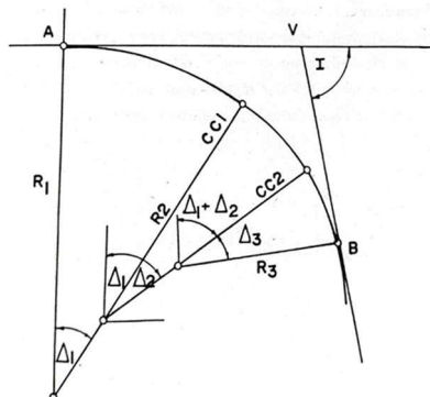
รูปภาพที่ ๓๒ โค้งผสมมี ๓ ศูนย์กลาง ที่มา: จิรพัฒน์ โชติกไกร. (๒๕๓๑).
