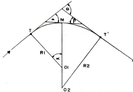
รูปภาพที่ ๓๑ โค้งผสมมี ๒ ศูนย์กลาง ที่มา: จิรพัฒน์ โชติกไกร. (๒๕๓๑).
