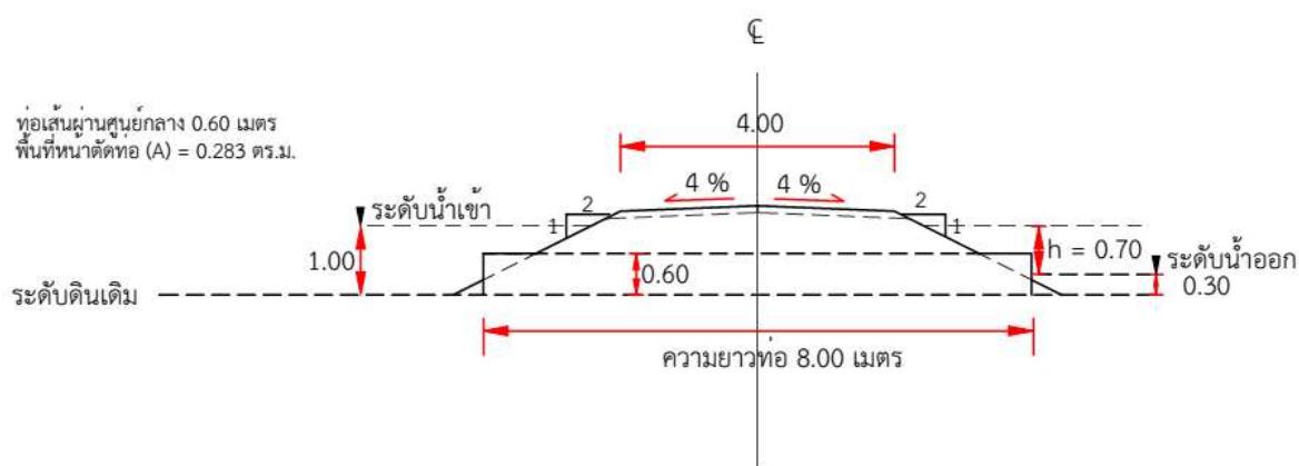
รูปภาพที่ ๙๕ ท่อ Ø ๐.๖๐ เมตร
