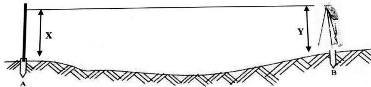
รูปภาพที่ ๒๖ การทำระดับโดยส่องไม้วัดระดับ (Staff) ที่หมุด A ที่มา: มานัส ยอดทอง.(ม.ป.ป.).
