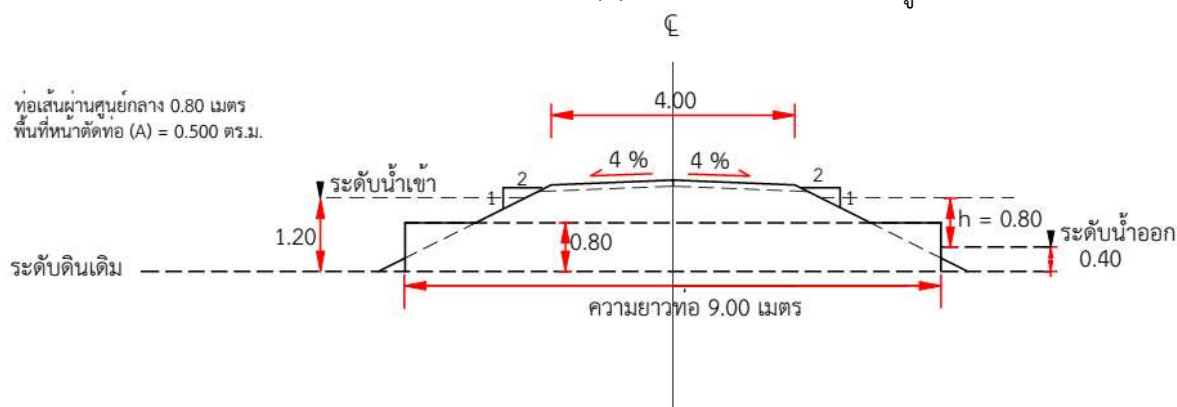
รูปภาพที่ ๙๖ ท่อ Ø ๐.๘๐ เมตร
