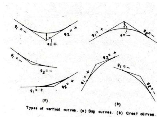
รูปภาพที่ ๓๗ ลักษณะต่าง ๆ ของโค้งตั้ง (a) โค้งหยาบ (b) โค้งคว่ำ ที่มา: จิรพัฒน์ โชติกไกร. (๒๕๓๑).
