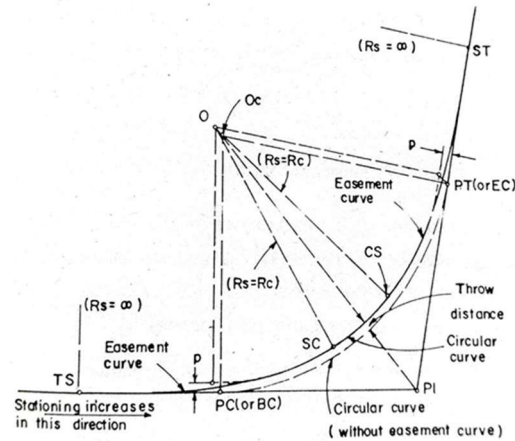
รูปภาพที่ ๓๕ แสดงการเชื่อมต่อระหว่างโค้งก้นหอยและโค้งวงกลม ที่มา: จิรพัฒน์ โชติกไกร. (๒๕๓๑).
