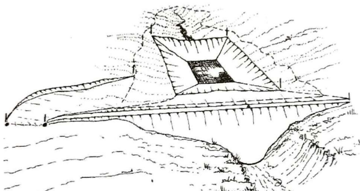
รูปภาพที่ ๕๕ สระเก็บน้ำในร่องน้ำตื้น ที่มา: สำนักงานการปฏิรูปที่ดินเพื่อเกษตรกรรม.(๒๕๖๑).
