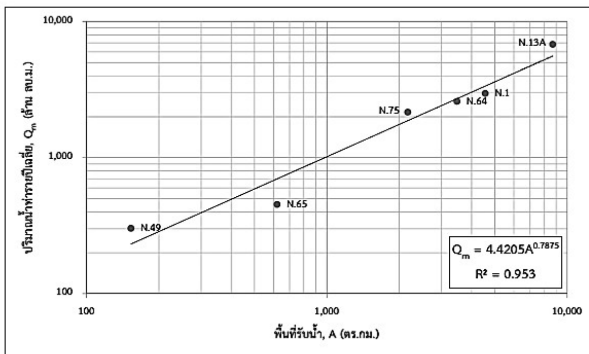
รูปภาพที่ ๒ ความสัมพันธ์ระหว่างปริมาณน้ำท่ารายปีเฉลี่ยกับขนาดพื้นที่รับน้ำของสถานีวัดน้ำท่าที่ตั้งอยู่ในอำเภอเมืองน่าน จังหวัดน่าน และบริเวณใกล้เคียง (ลุ่มน่านตอนบน) ที่มา: โครงการศึกษาจัดทำแผนแม่บทการพัฒนาแหล่งน้ำและระบบกระจายน้ำในเขตปฏิรูปที่ดิน จังหวัดแพร่ น่าน และอุดรดิตถ์ (๒๕๖๔)
