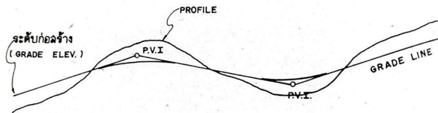
รูปภาพที่ ๓๖ ทางขึ้นและลงเนินที่ต้องออกแบบโค้งทางตั้ง ที่มา: จิรพัฒน์ โชติกไกร. (๒๕๓๑).
