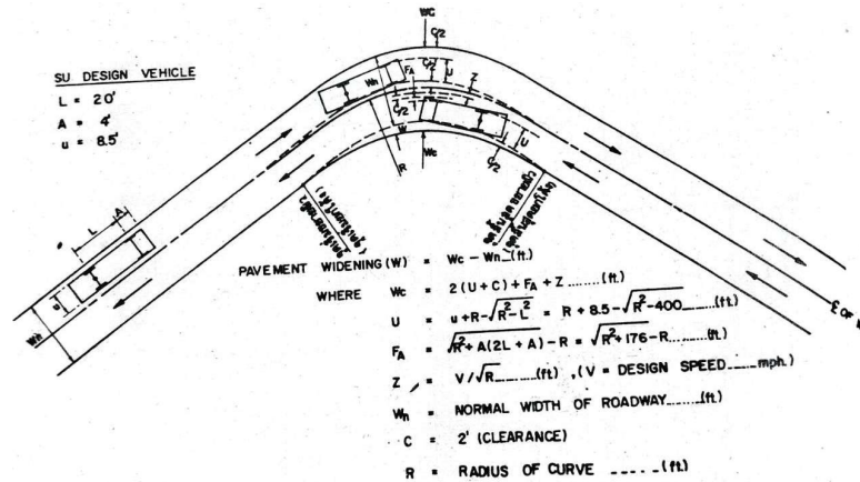
รูปภาพที่ ๔๕ การขยายขอบทางโค้งตามวิธีของ AASHTO ที่มา: จิรพัฒน์ โชติกไกร. (๒๕๓๑).
