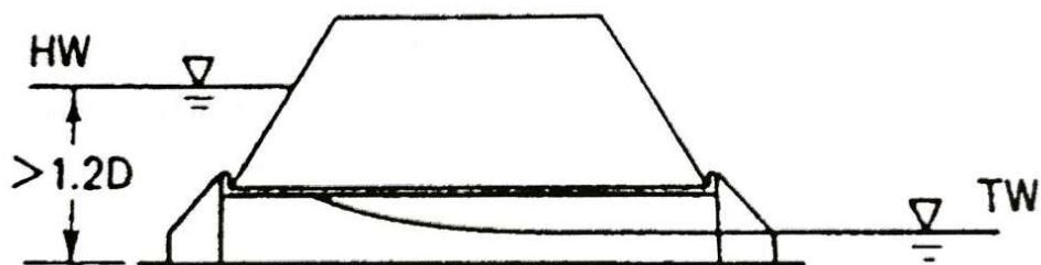
รูปภาพที่ ๕๗ ท่อลอดทางเข้าจมนและทางออกไม่จมนเป็นการไหลแบบรูระบาย ที่มา: สำนักงานการปฏิรูปที่ดินเพื่อเกษตรกรรม.(๒๕๖๑).
