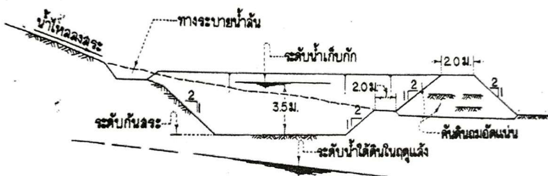
รูปภาพที่ ๕๔ รูปตัดตามยาว
