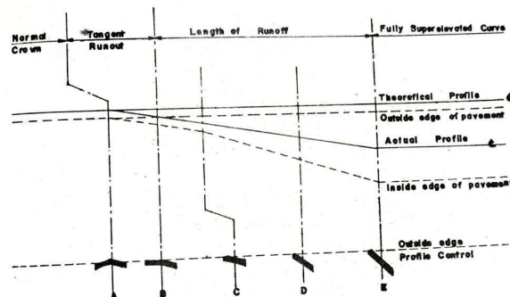
รูปภาพที่ ๔๓ การยกขอบทางโค้งใช้ขอบถนนด้านนอกเป็นจุดหมุน ที่มา: จิรพัฒน์ โชติกไกร. (๒๕๓๑).
